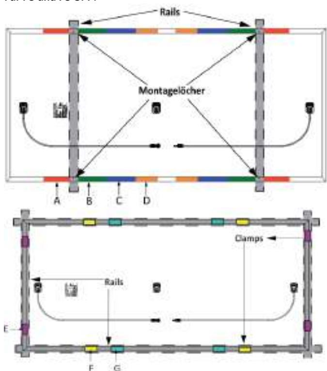
Abbildung 4: Klemmbereich für die Module der Performance Serie
