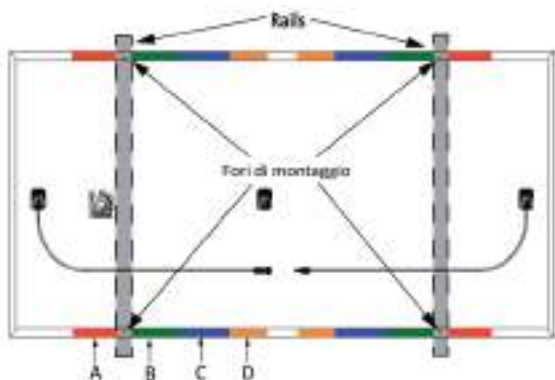
Figura 4: Zone di montaggio delle delle pinze o morsetti per il modulo Performance UPP
