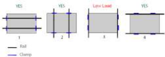
図 3. 架台の構成
