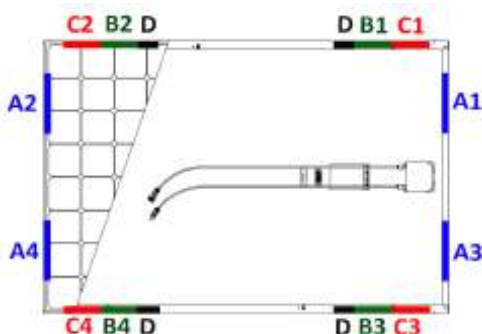
Abbildung 2: Befestigungszonen für Maxeon Module
