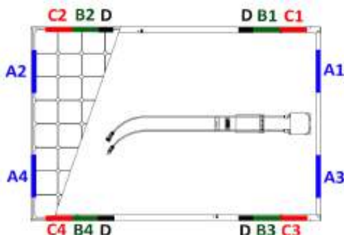
Figura 2: zone di montaggio delle delle pinze o morsetti per il modulo Maxeon
